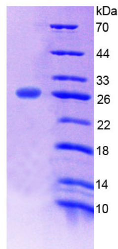
15% SDS-PAGE
