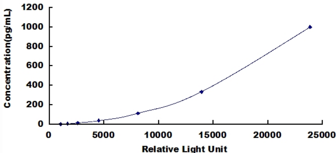
人轻肽神经丝蛋白 (NEFL) 检测试剂盒标准曲线
