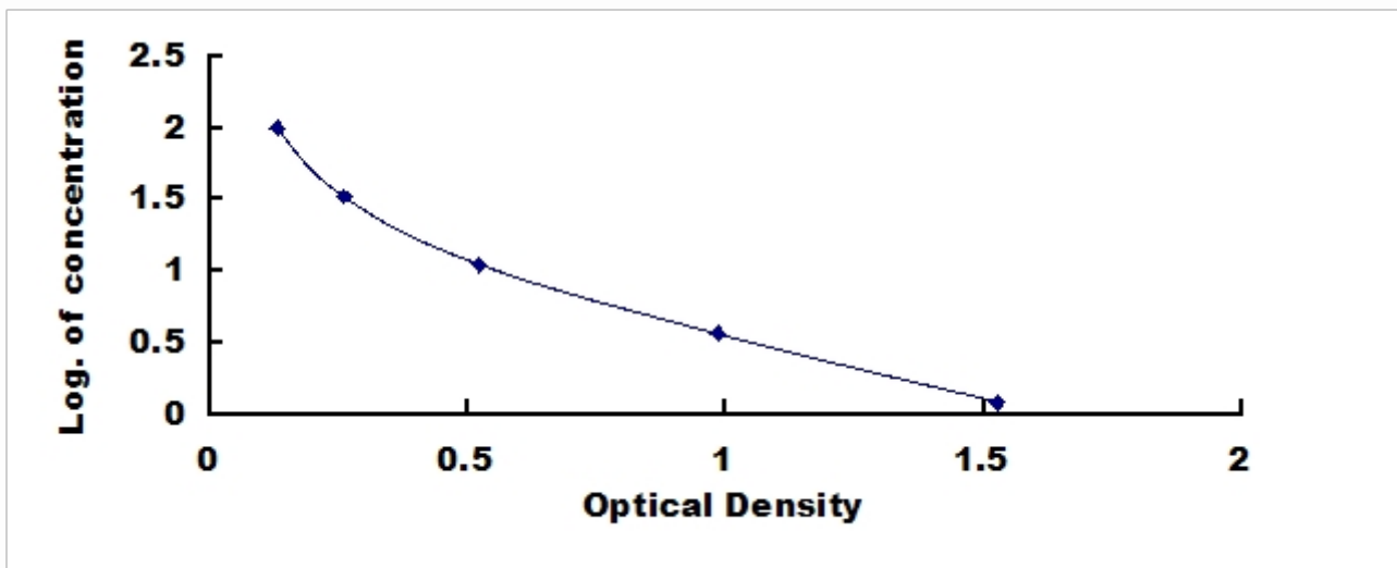
2,3-二磷酸甘油酸(2,3-BPG)检测试剂盒标准曲线
