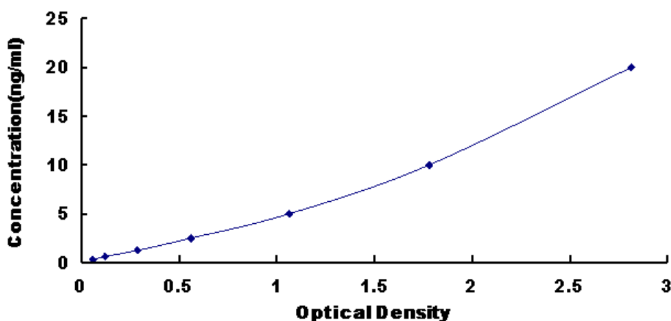
图 1: 人的解整合素样金属蛋白酶 17(ADAM17)试剂盒标准曲线
