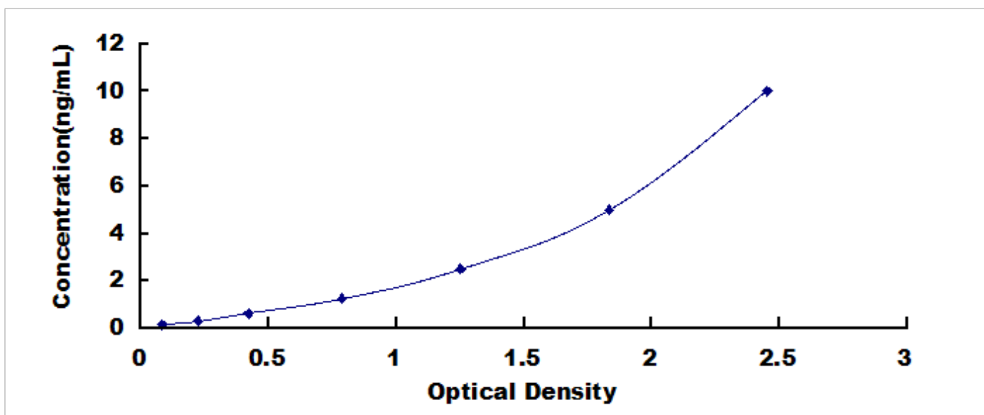
人 ATP 结合盒转运蛋白 A1 (ABCA1) 检测试剂盒标准曲线
