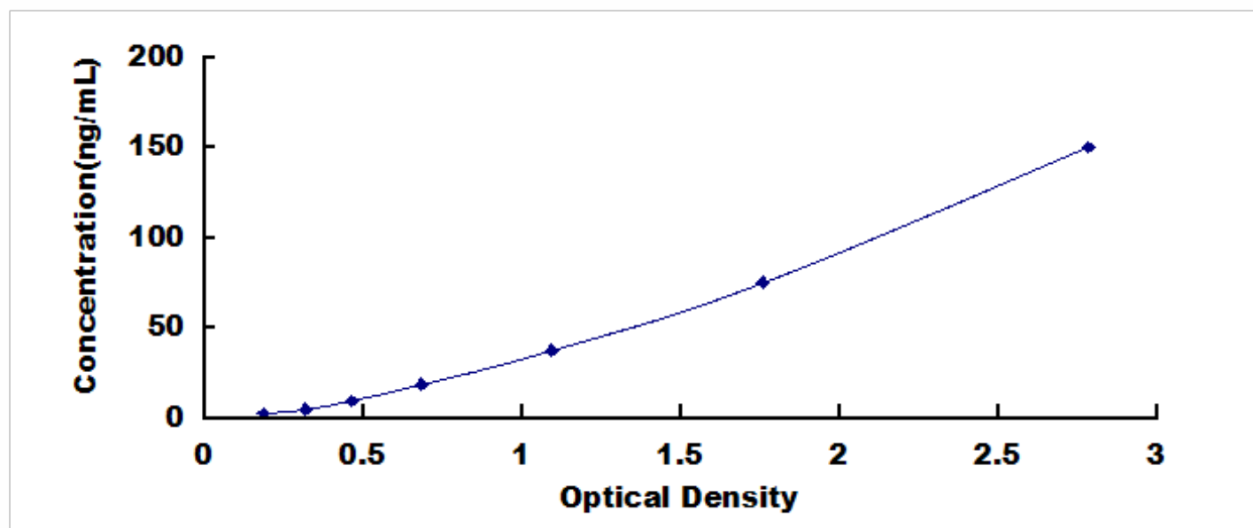
大鼠 AXL 受体酪氨酸激酶(AXL)检测试剂盒标准曲线
