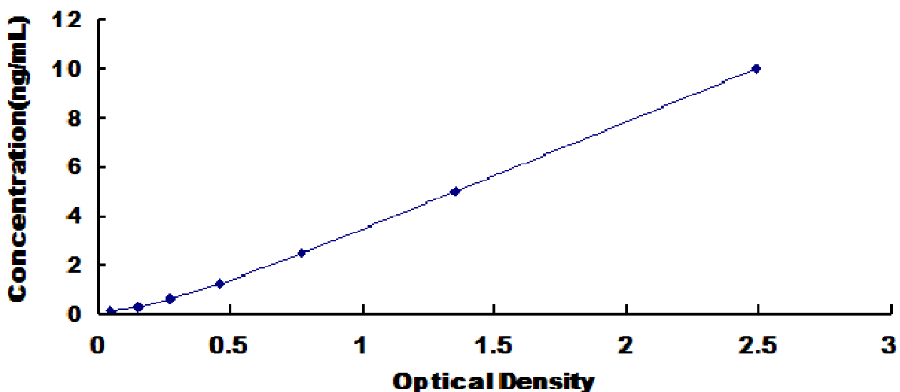
人 Ab1 交互子 1 (ABI1) 检测试剂盒标准曲线
