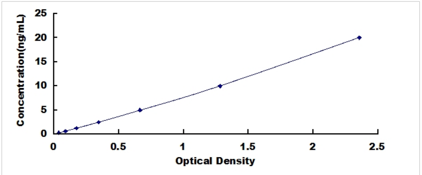
人 Ab1 相互作用蛋白 3 (ABI3) 检测试剂盒标准曲线
