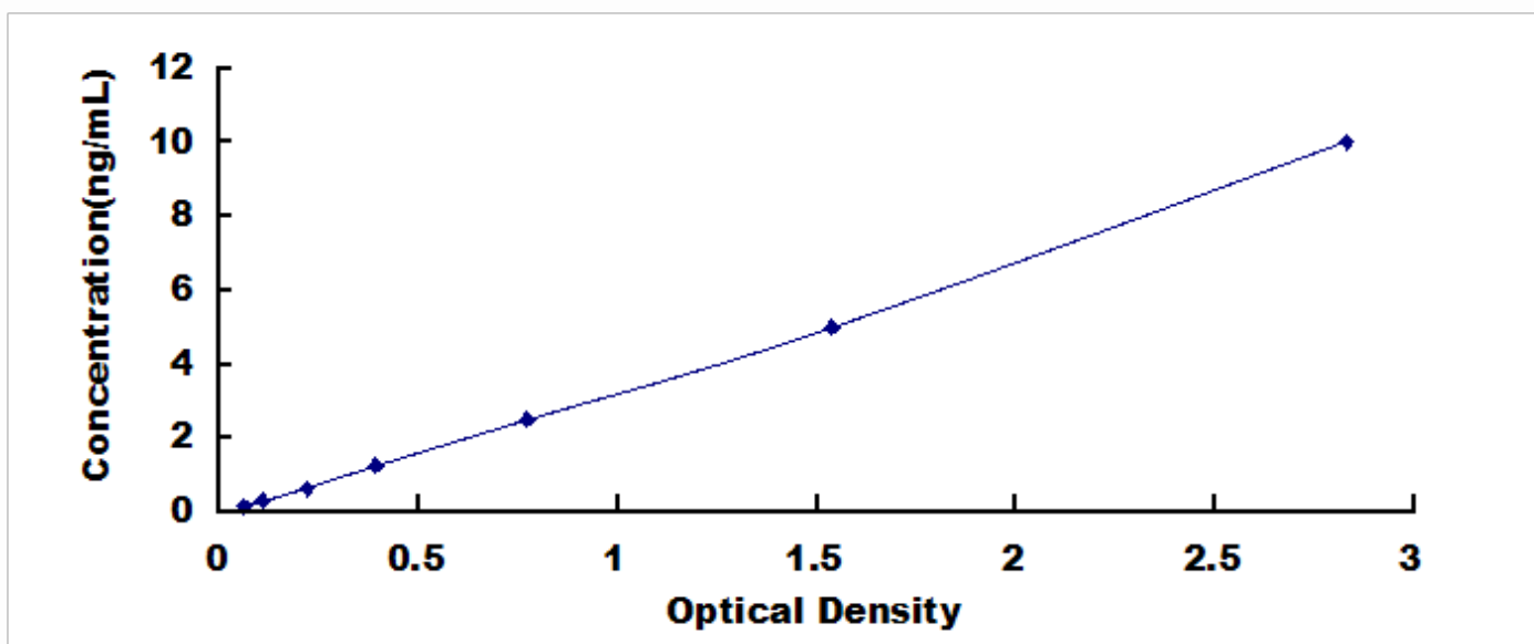
小鼠乙酰辅酶 A 乙酰转移酶 1 (ACAT1) 检测试剂盒标准曲线
