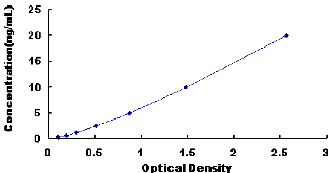
小鼠乙酰辅酶 A 羧化酶 \alpha (ACAC \alpha ) 试剂盒标准曲线
