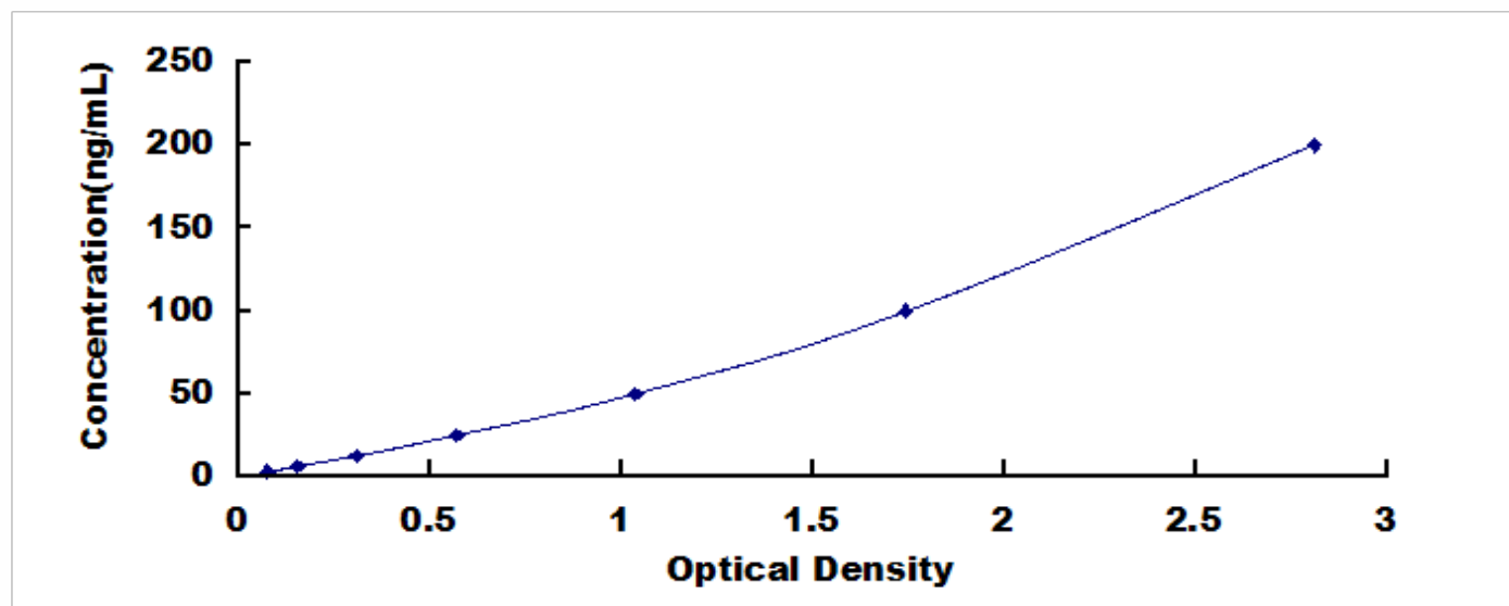
大鼠乙酰胆碱酯酶(AchE)检测试剂盒标准曲线
