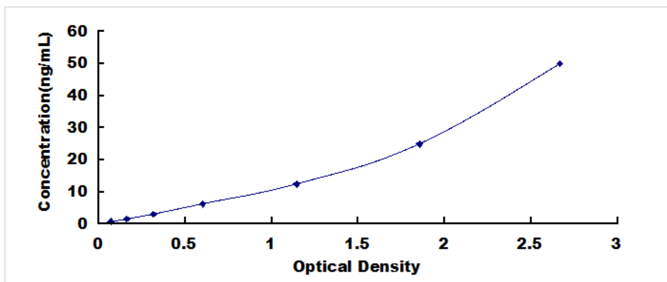
大鼠抗酒石酸酸性磷酸酶(ACP5)检测试剂盒标准曲线
