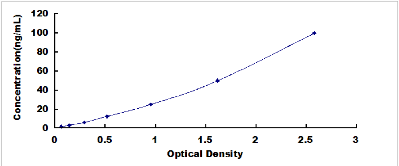
肌动蛋白 β (ACT β) 检测试剂盒标准曲线
