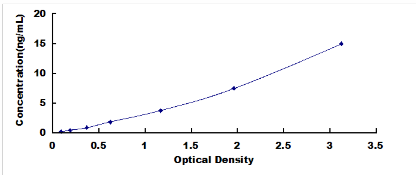
人极低密度脂蛋白 (VLDL) 检测试剂盒标准曲线
