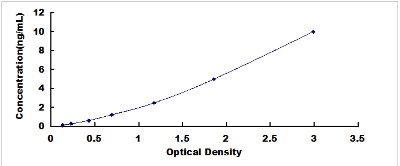
人腺苷高半胱氨酸水解酶(AHCY)检测试剂盒标准曲线
