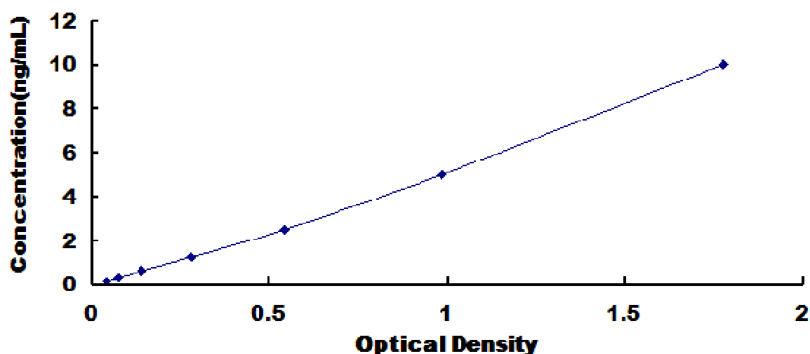
大鼠肾上腺素能受体 \beta 1 (ADR \beta 1) 检测试剂盒标准曲线
