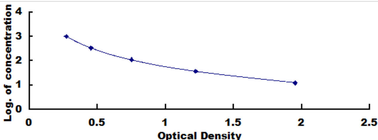
人肾上腺髓质素 (ADM) 检测试剂盒标准曲线
