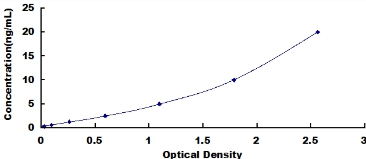
大鼠聚集蛋白聚糖 (AGC) 检测试剂盒标准曲线
