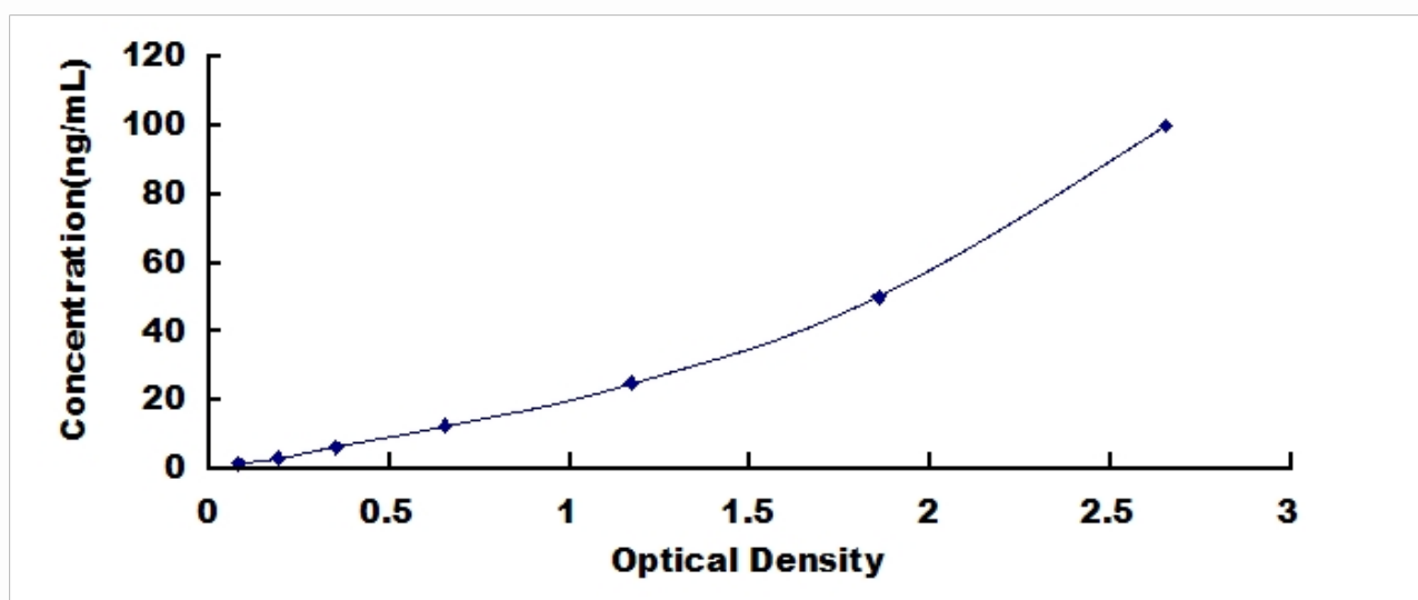
人丙氨酸乙醛酸转氨酶 (AGXT) 检测试剂盒标准曲线
