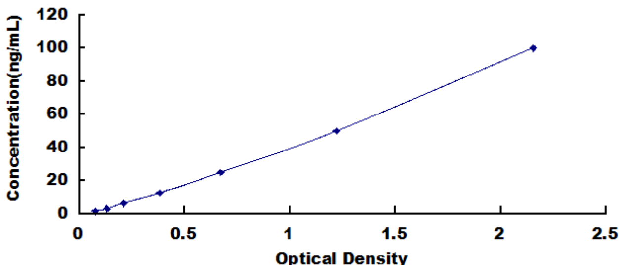
小鼠醛脱氢酶 1 家族成员 A1 (ALDH1A1) 检测试剂盒标准曲线
