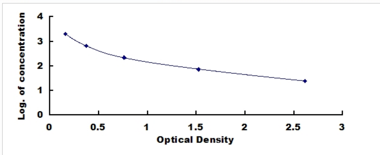
醛固酮 (ALD) 检测试剂盒标准曲线
