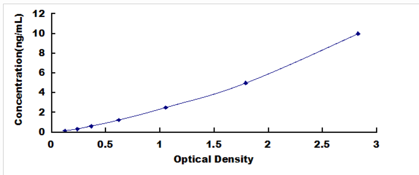
小鼠碱性磷酸酶(ALP)检测试剂盒标准曲线
