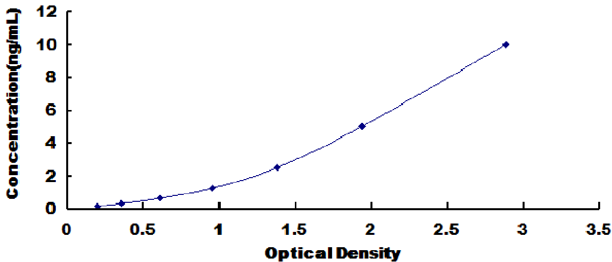
牛碱性磷酸酶 (ALP) 检测试剂盒标准曲线
