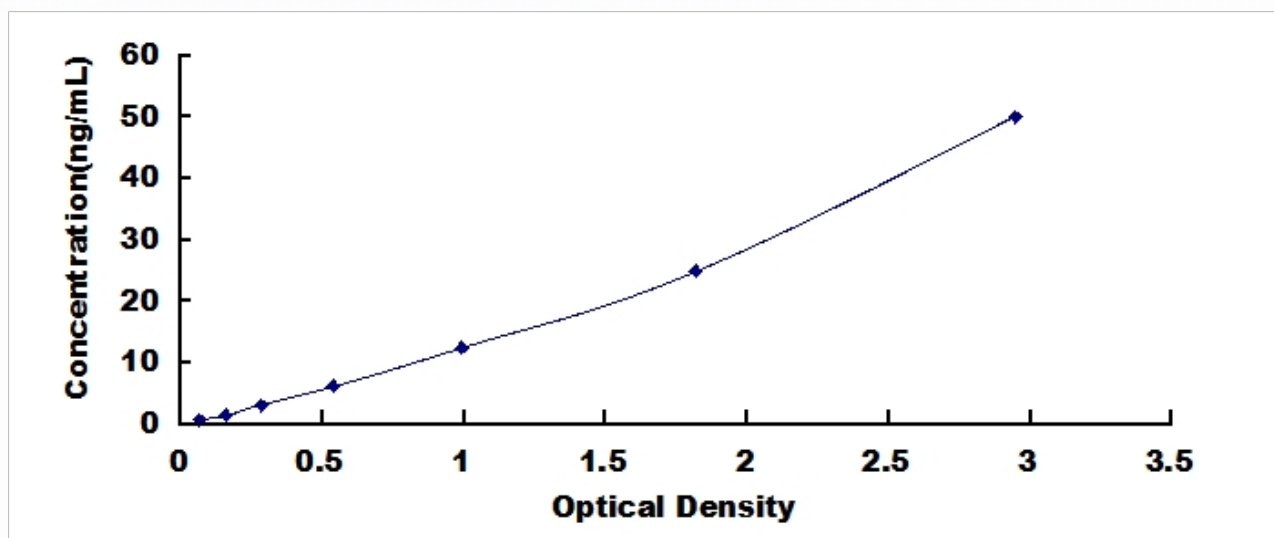
大鼠肝肾骨碱性磷酸酶(ALPL)检测试剂盒标准曲线
