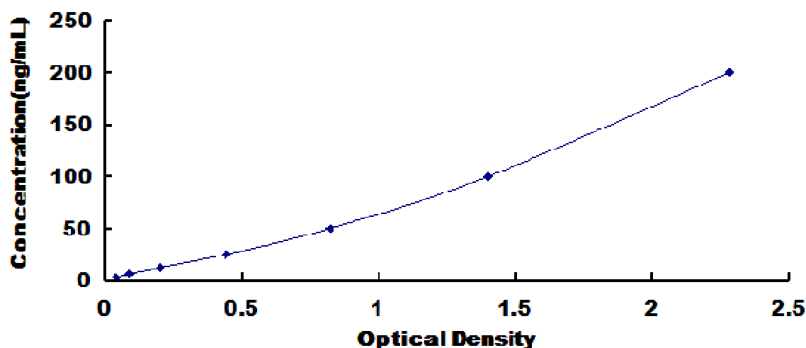
人碱性鞘磷脂磷酸二酯酶(Alk-Smase)检测试剂盒标准曲线
