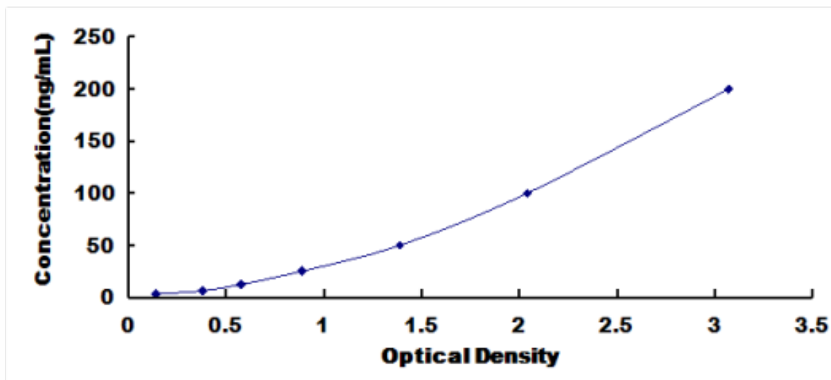
人 \alpha 1 -抗胰蛋白酶 ( \alpha 1AT ) 检测试剂盒标准曲线
