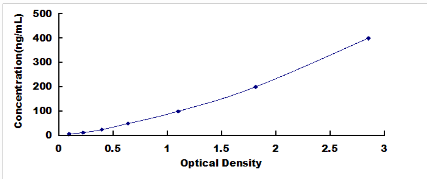
人 \alpha 1-抗胰蛋白酶 ( \alpha 1AT) 检测试剂盒标准曲线
