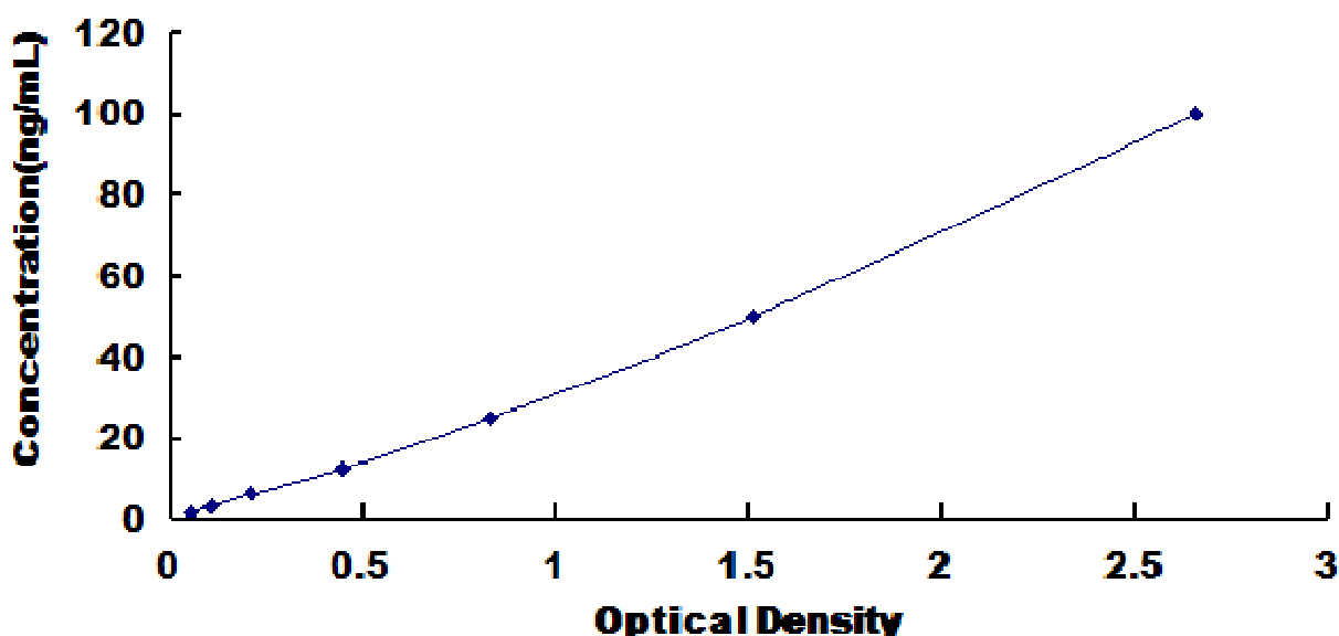
人 \alpha 1B 糖蛋白( \alpha 1BG)试剂盒标准曲线
