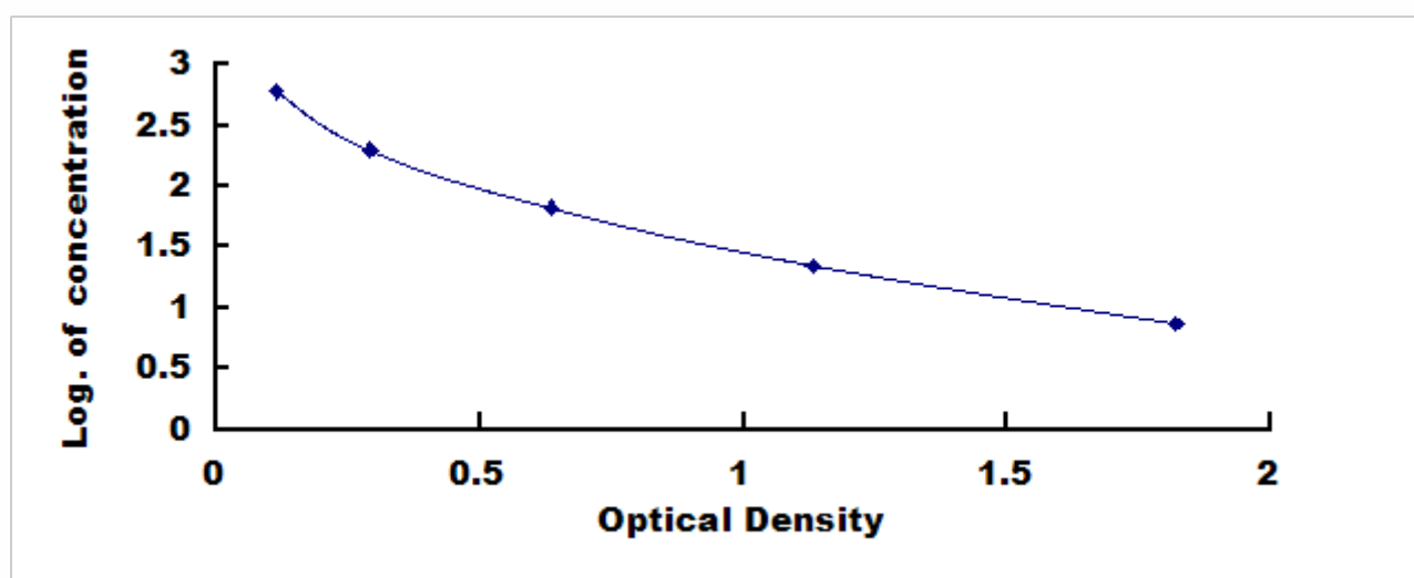
小鼠 \alpha 2-巨球蛋白 ( \alpha 2M) 检测试剂盒标准曲线
