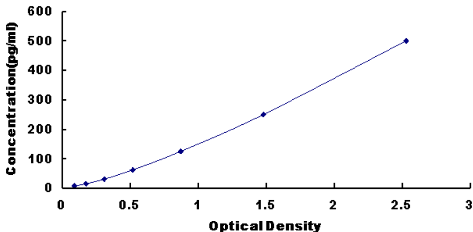
图 1: 人的双调蛋白(AR)试剂盒标准曲线
