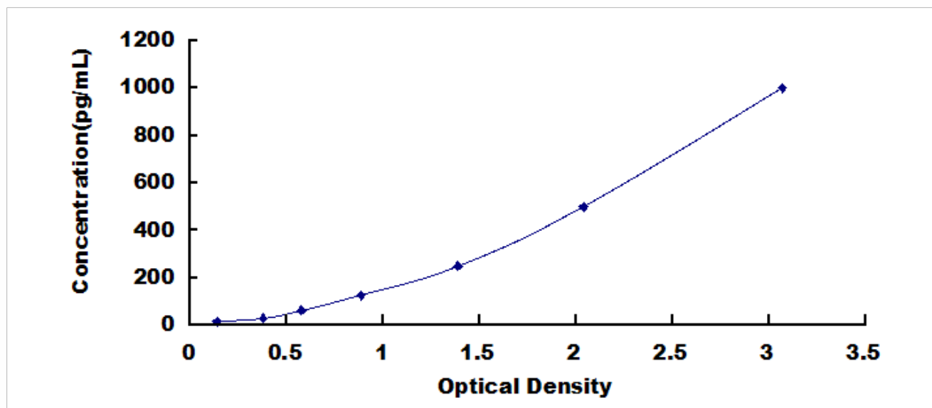
小鼠淀粉样蛋白 \beta 1-42 (A \beta 1-42) 检测试剂盒标准曲线
