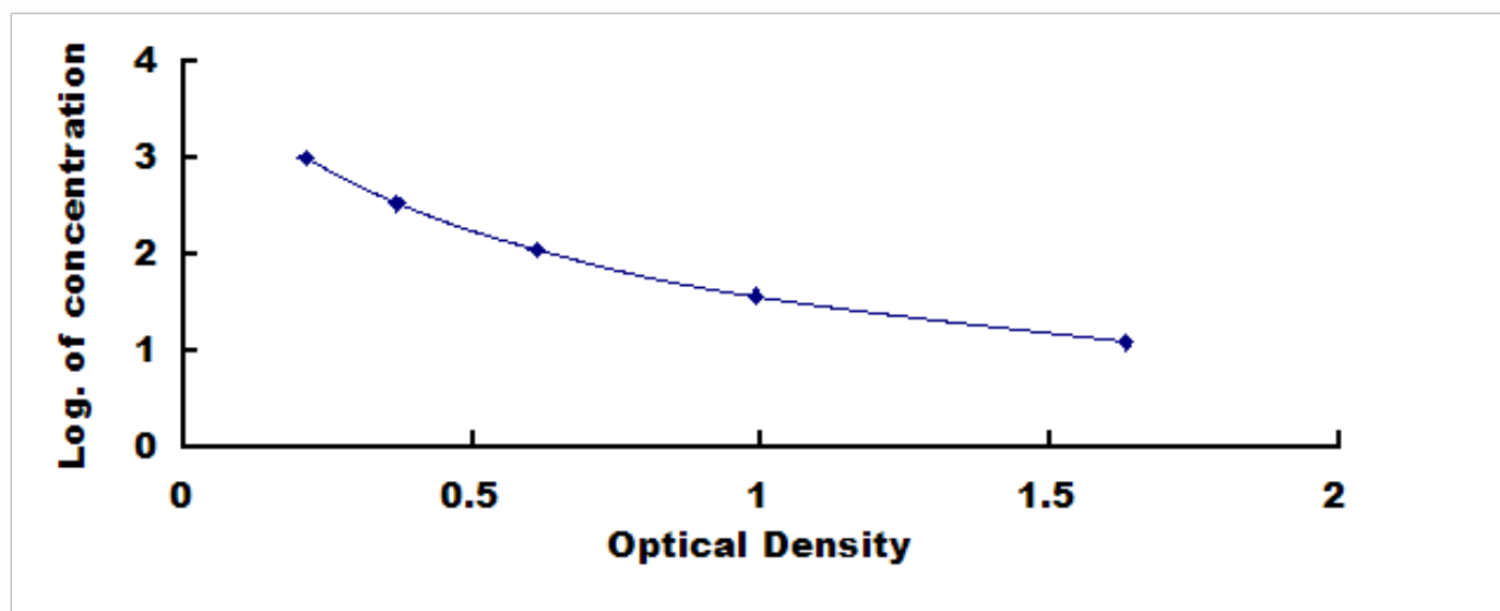
大鼠淀粉样蛋白 \beta 1-42 (A \beta 1-42) 检测试剂盒标准曲线
