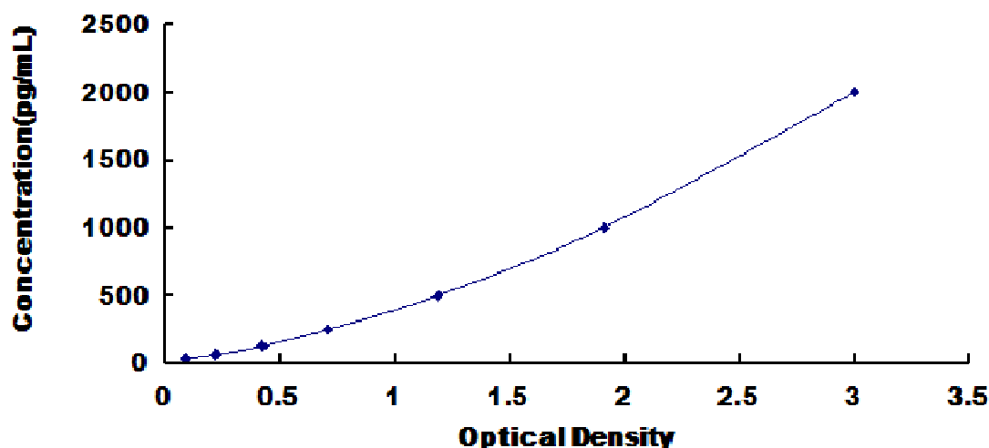
人血管生长素(ANG)检测试剂盒标准曲线
