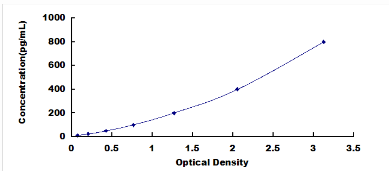
大鼠血管生成素 2 (ANGPT2) 检测试剂盒标准曲线
