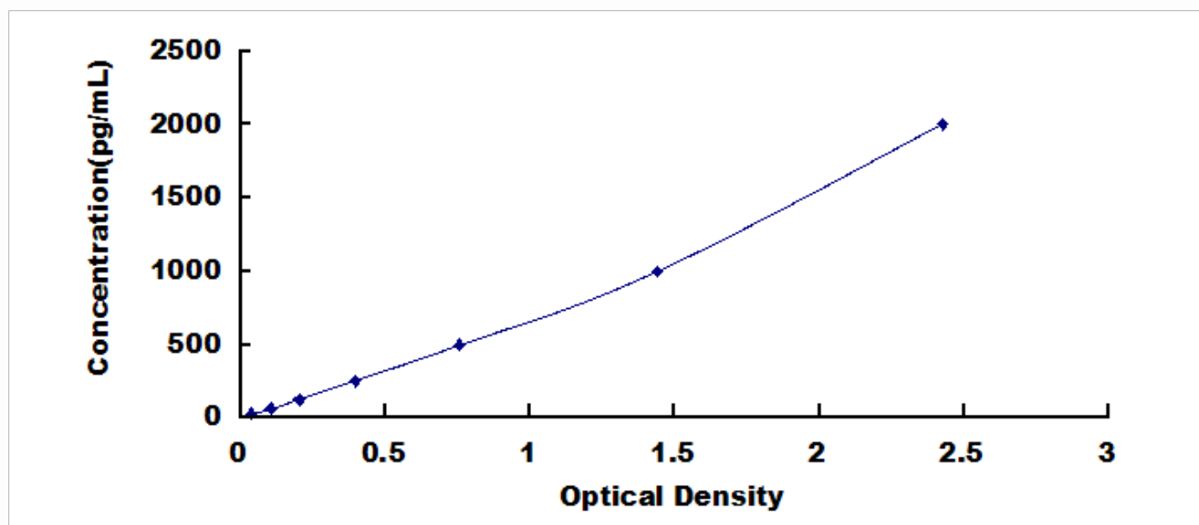
小鼠血管生成素样蛋白 2 (ANGPTL2) 检测试剂盒标准曲线
