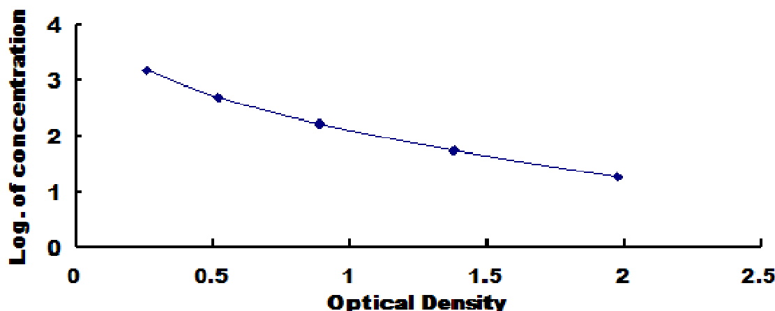
人血管紧张素 1-9(Ang1-9)检测试剂盒标准曲线
