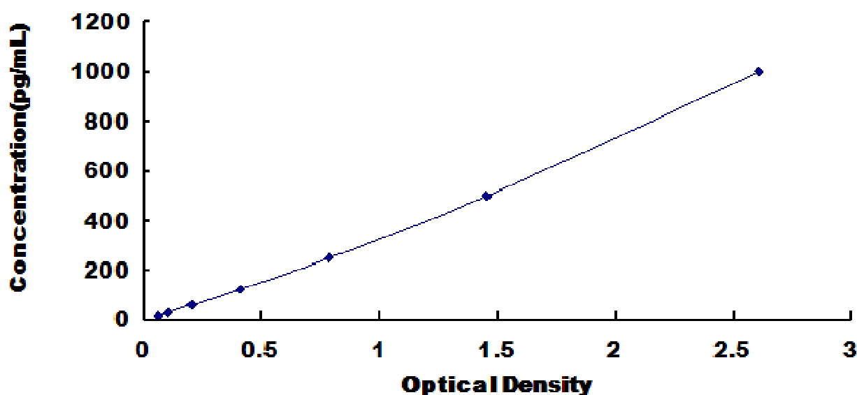
人血管紧张素转化酶 2 (ACE2) 检测试剂盒标准曲线
