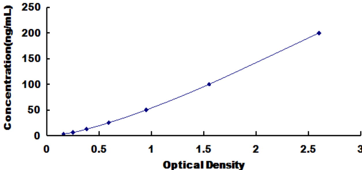
人抗甘露糖结合蛋白抗体(Anti-MBL)试剂盒标准曲线
