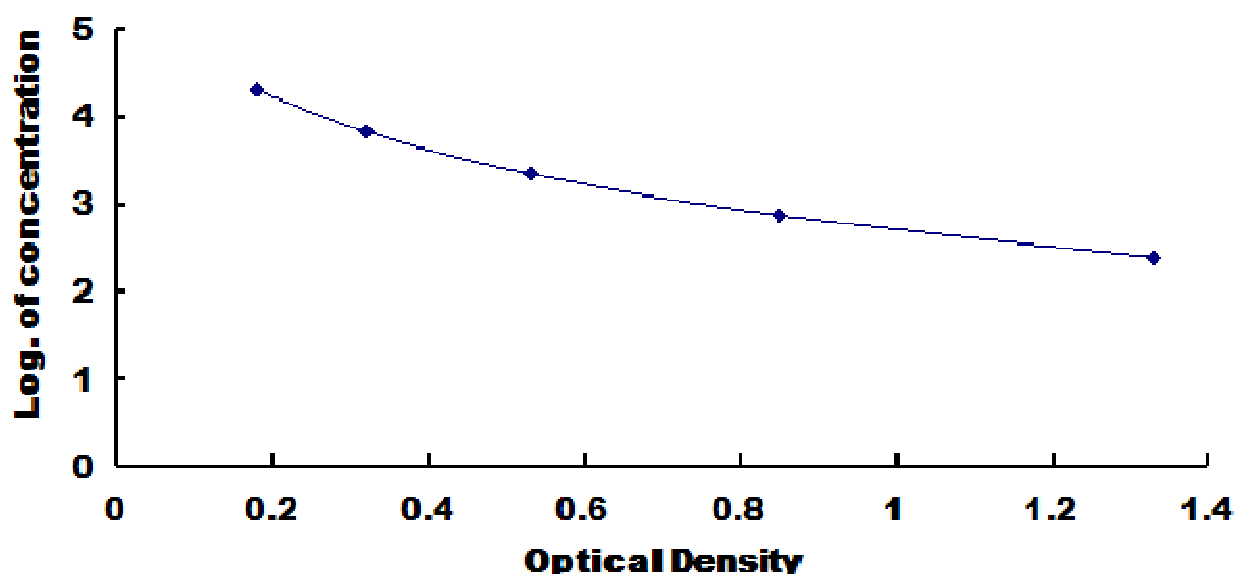
小鼠抗缪勒管激素(AMH)试剂盒标准曲线
