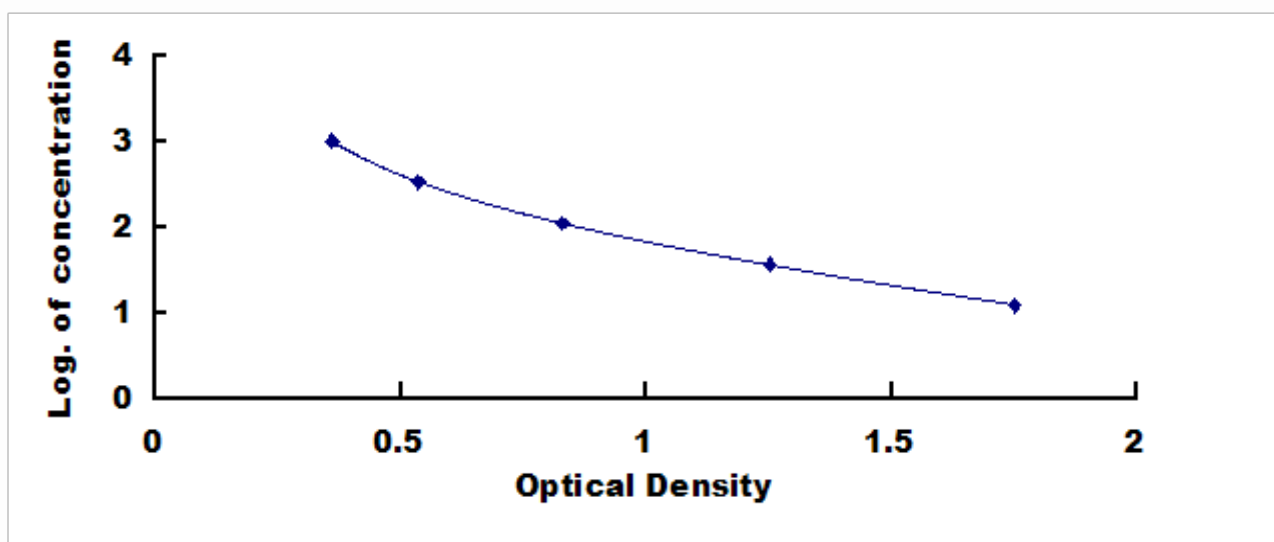
人抗利尿激素 (ADH) 检测试剂盒标准曲线
