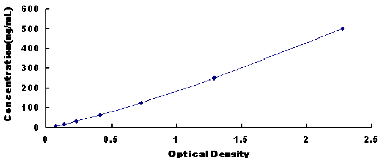
大鼠载脂蛋白 A4 (APOA4) 试剂盒标准曲线
