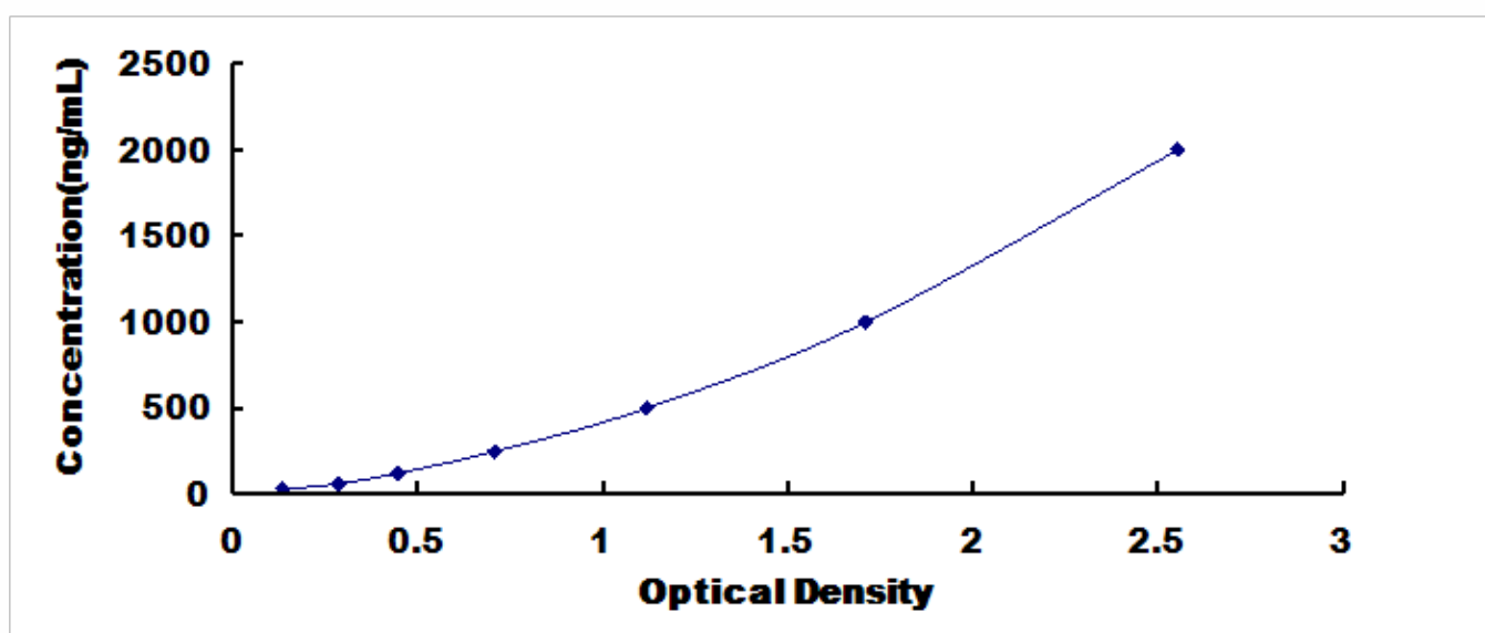
大鼠载脂蛋白 B (APOB) 检测试剂盒标准曲线
