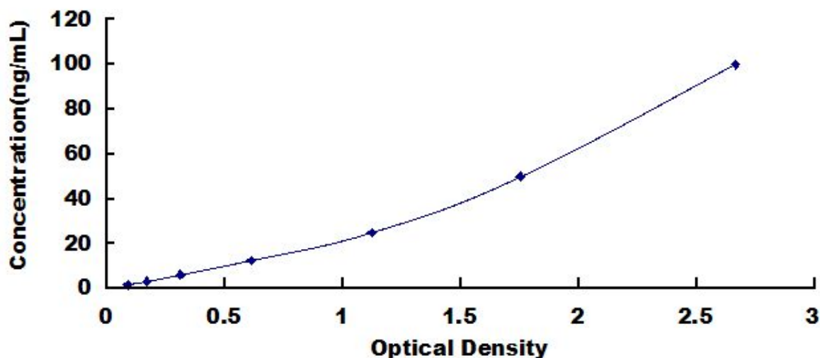
人载脂蛋白 C2 (APOC2) 检测试剂盒标准曲线
