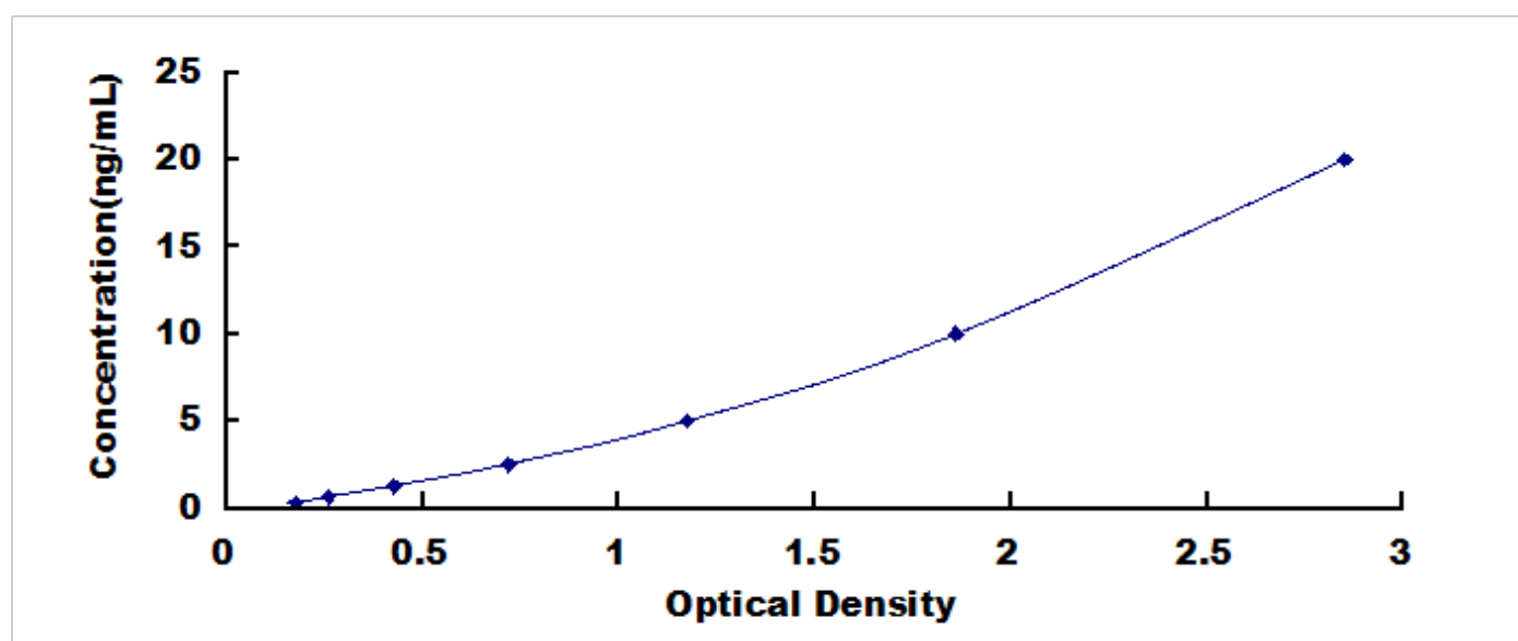
人载脂蛋白 C3 (APOC3) 检测试剂盒标准曲线
