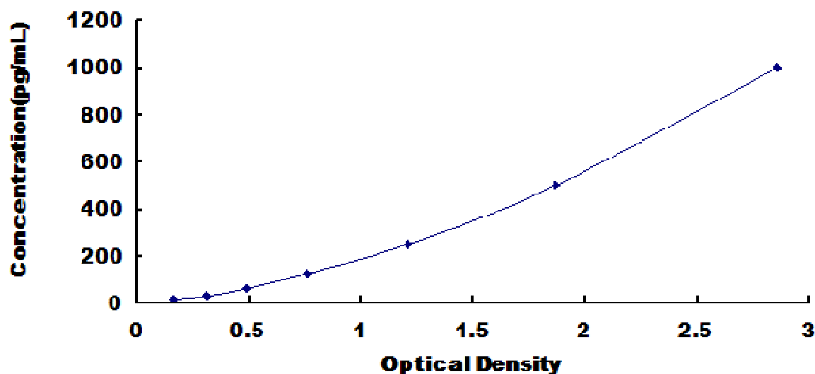
人抑制蛋白 \beta 2 (ARR \beta 2) 检测试剂盒标准曲线
