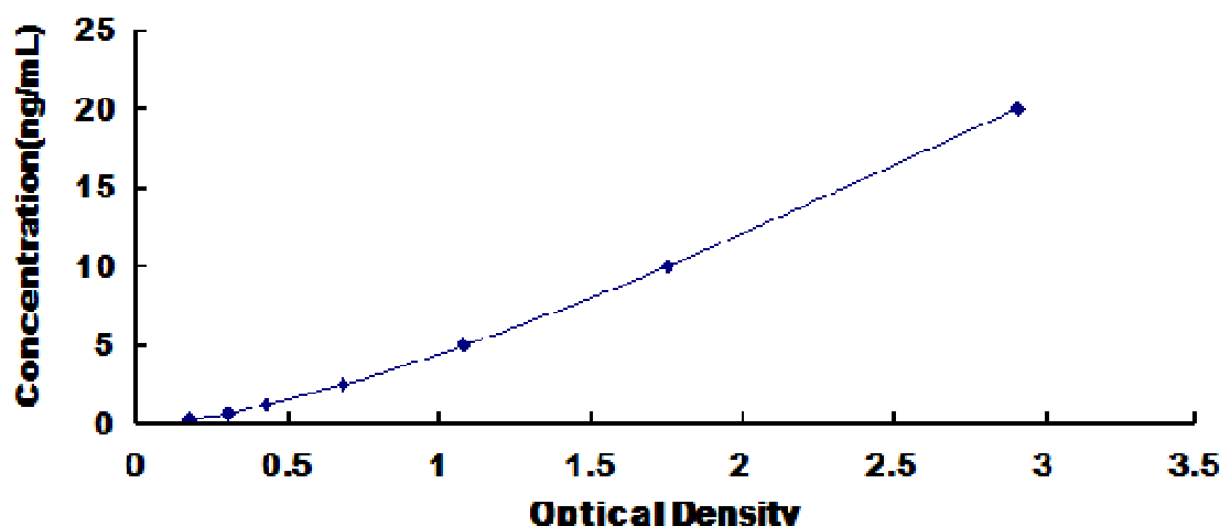
人芳香烃受体(AhR)试剂盒标准曲线
