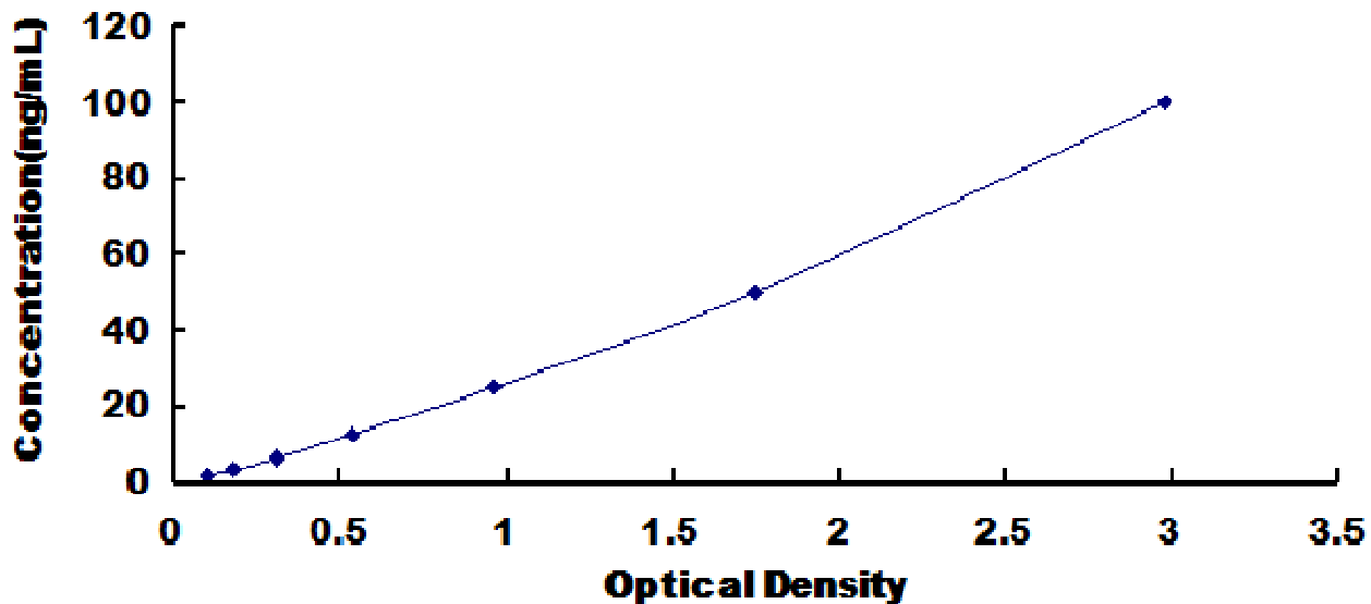
人芳犬尿氨酸甲酰胺酶(AFMID)检测试剂盒标准曲线
