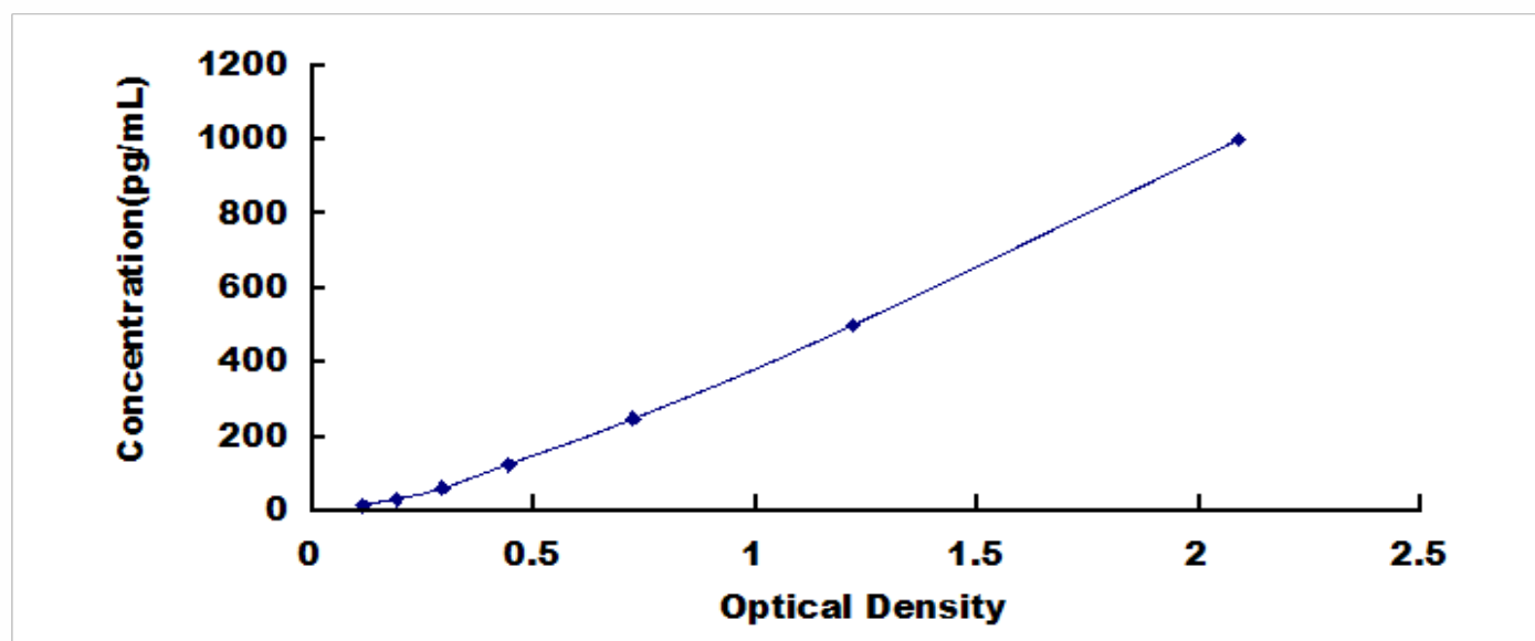
人心钠肽 (ANP) 检测试剂盒标准曲线
