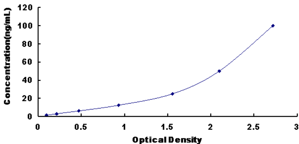
图 1: 大鼠 \beta 2 微球蛋白( \beta 2M )试剂盒标准曲线
