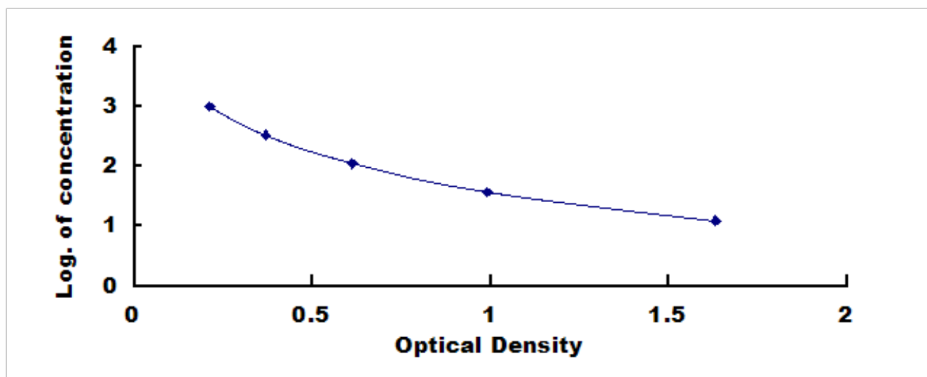
大鼠 \beta -内啡肽 ( \beta EP) 检测试剂盒标准曲线
